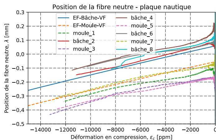
Figure 8: Comparaison entre expérimental et modèles bâche (EF-Bâche-VF) et moule (Ef-Moule-VF) intégrant les variations locales de taux de fibre.
