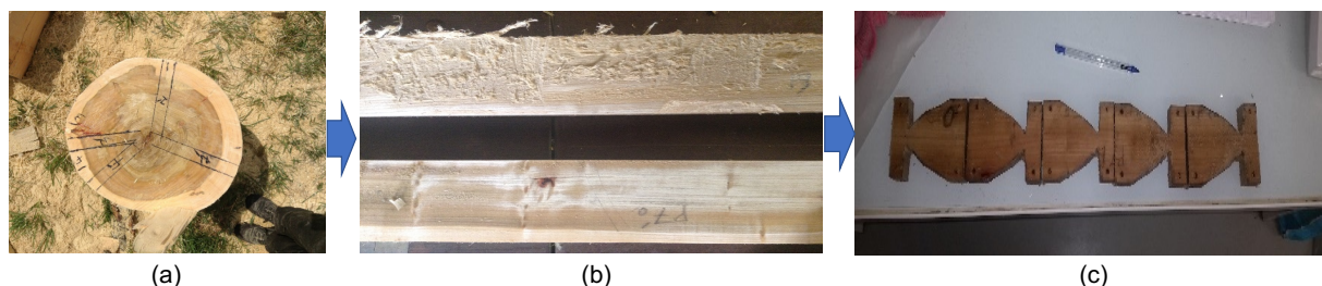
Figure 1 : (a) troncs haut du peuplier, (b) planches débitées, (c) éprouvettes MMCG
