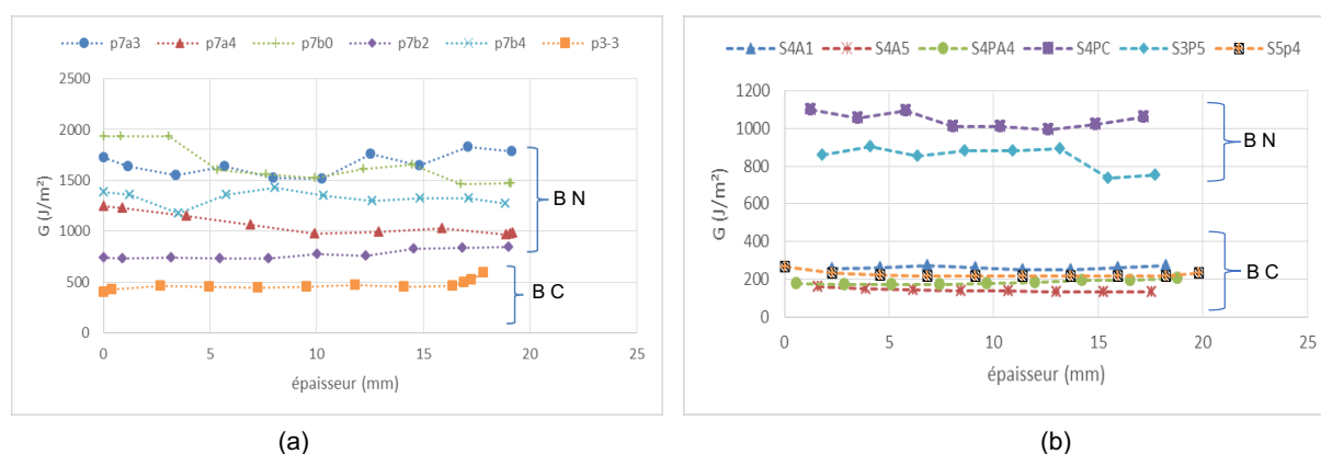
Figure 6 : évolution de G vs. position dans l'épaisseur : (a) peuplier ; (b) sapin.
