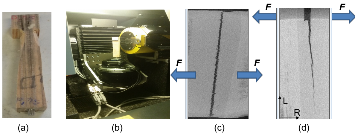
Figure 2 : échantillon : (a) Défilé ; (b) pour scan \mu CT ; (c) dans le scanner ; Observation de la fissure selon les plans RT (e) et RL (f).
